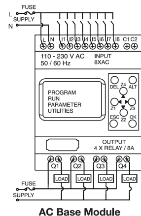
AC Base Module
