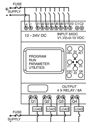
DC Base Module
